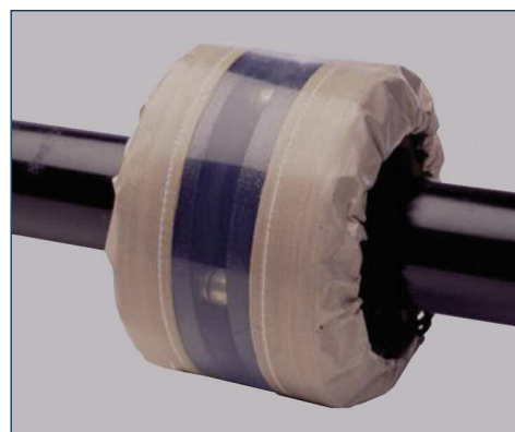
PTFE renforcé tissu de verre avec bande transparente en ECTFE
