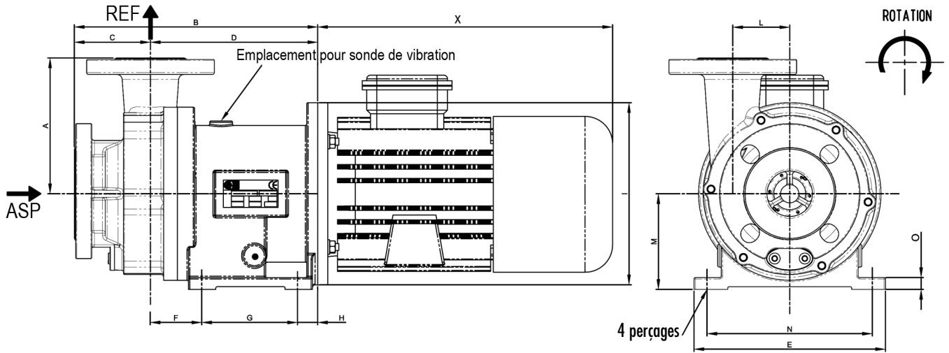
DIMENSIONS POMPE/MOTEUR(en mm)
